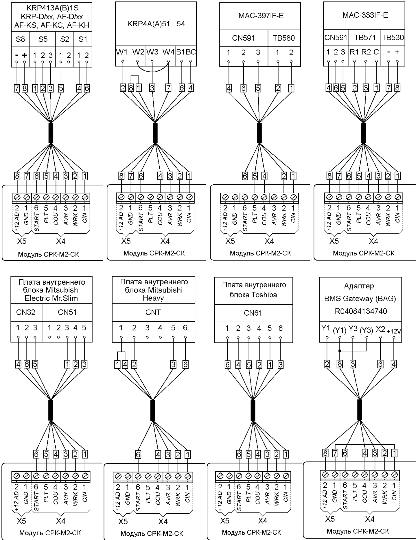
Рисунок 4.5 – Типовые схемы подключения СРК-М2-СК
