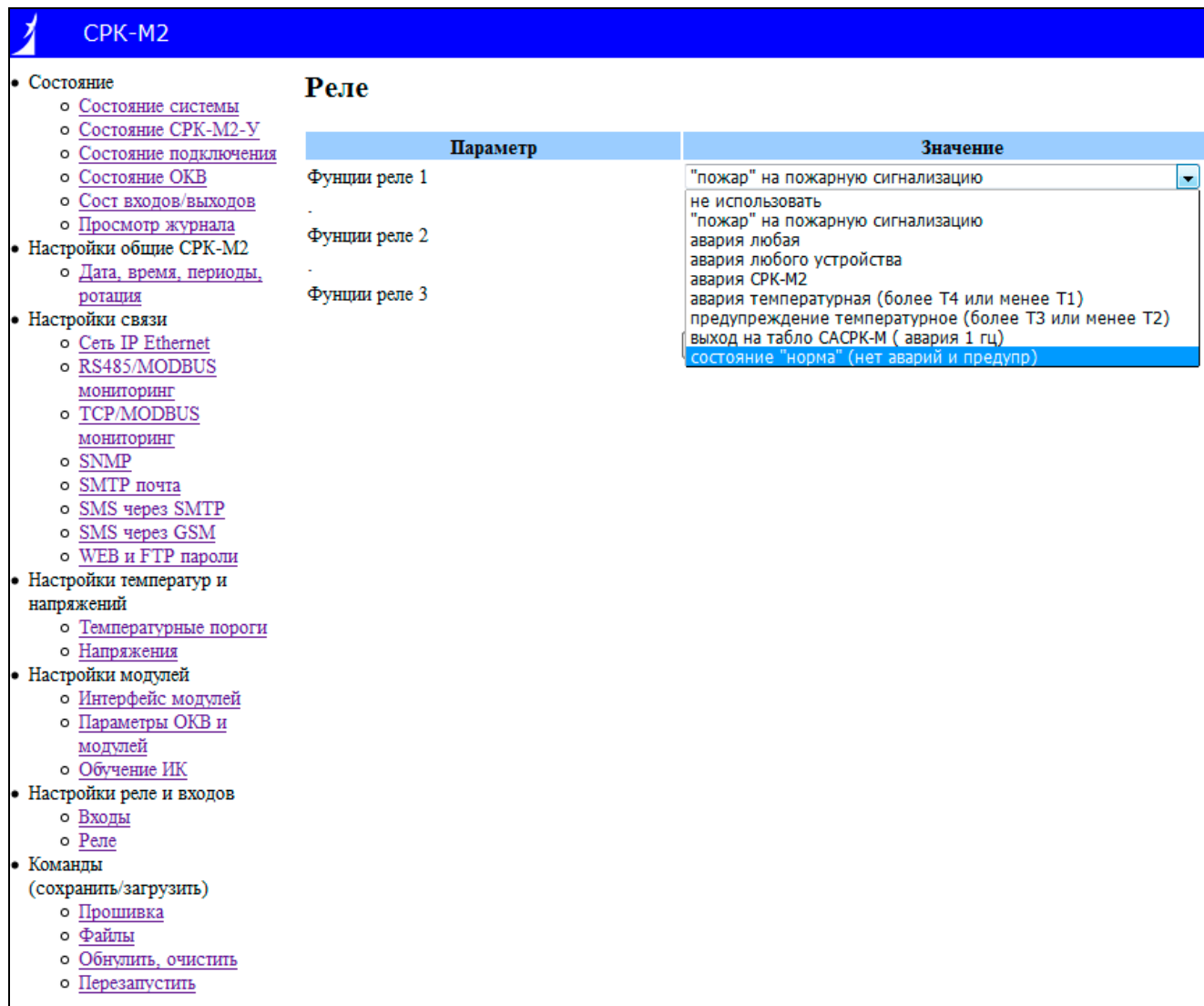
Рисунок 4.11 – Меню функций реле
