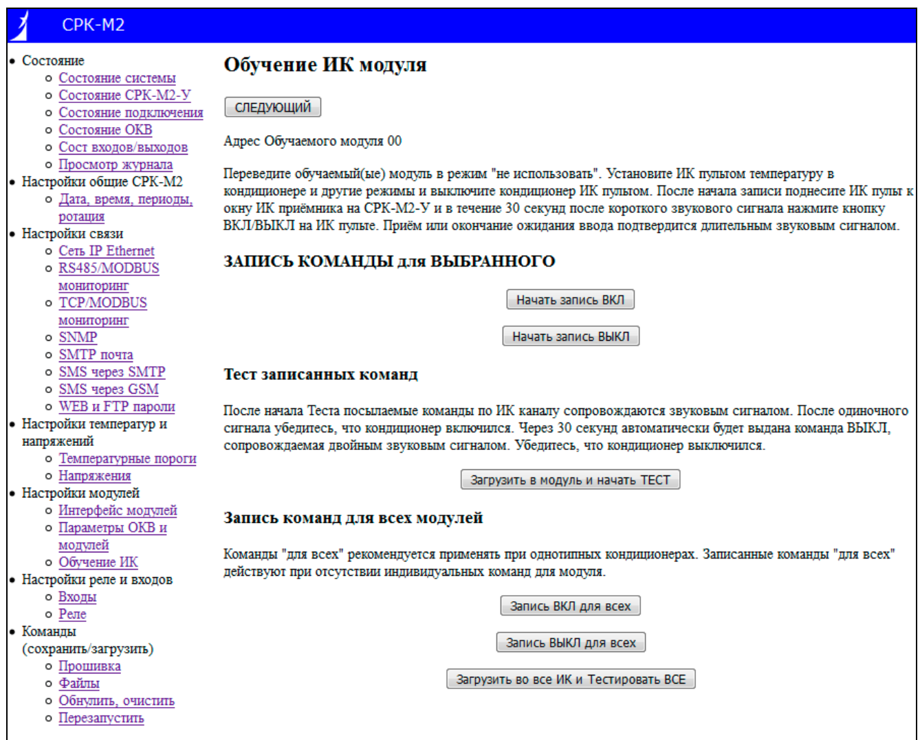
Рисунок 5.5 – Меню обучения ИК модуля
