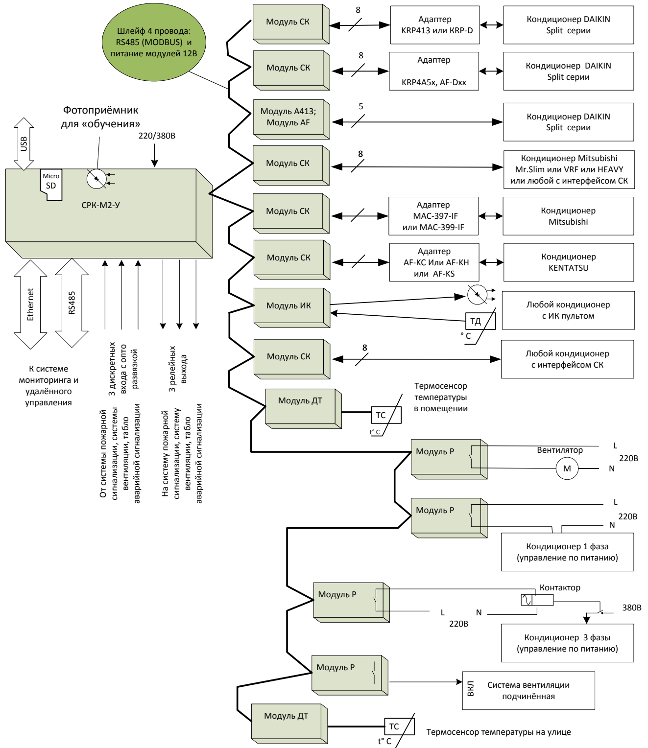
Рисунок 2.1- Структурная схема системы на базе СРК-М2
